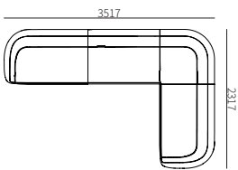
D02ZH-4 3517*2317*810mm 138.5*91.2*31.9"
