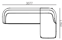
D02ZH-2 3077*1760*810mm 121.1*69.3*31.9"
