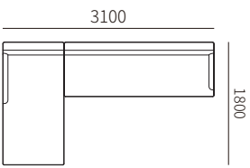
F52CR + F52A-2L 3100*1800*800MM 122.0*70.9*31.5"
