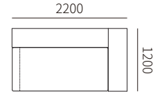
DA04C-2R 2200*1200*590MM 86.6*47.2*23.2"
